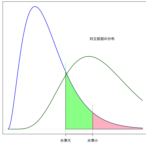
図 3: 検定の設計
