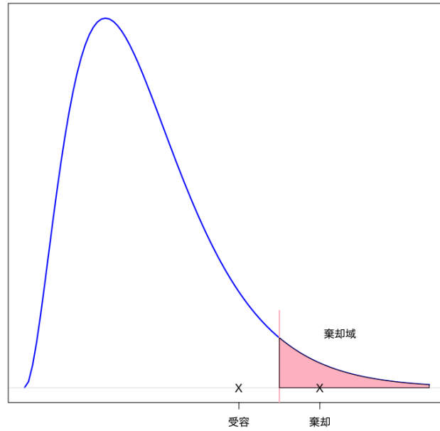
図 2: 棄却と受容
