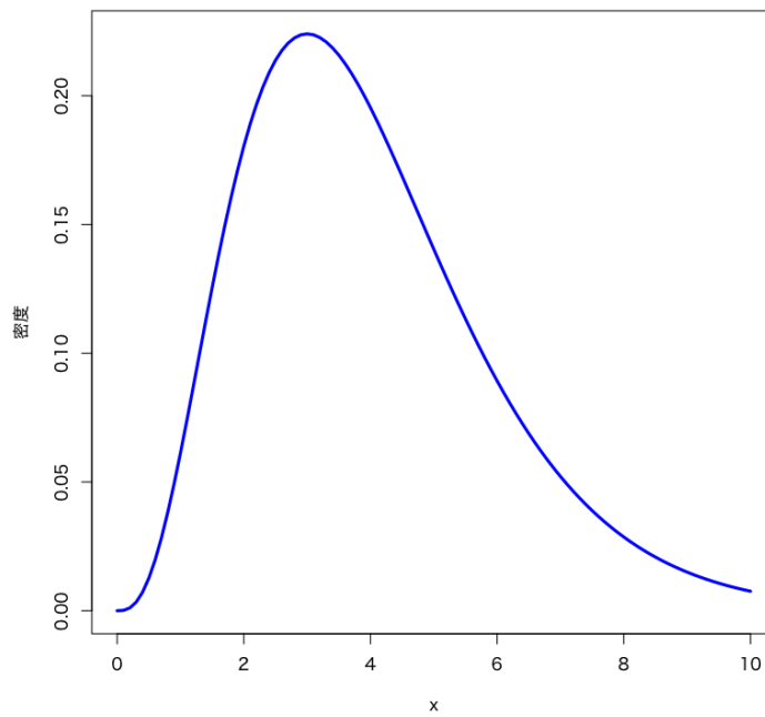
Gamma分布 (形状4, レート1; 歪度1, 超過尖度1.5)
