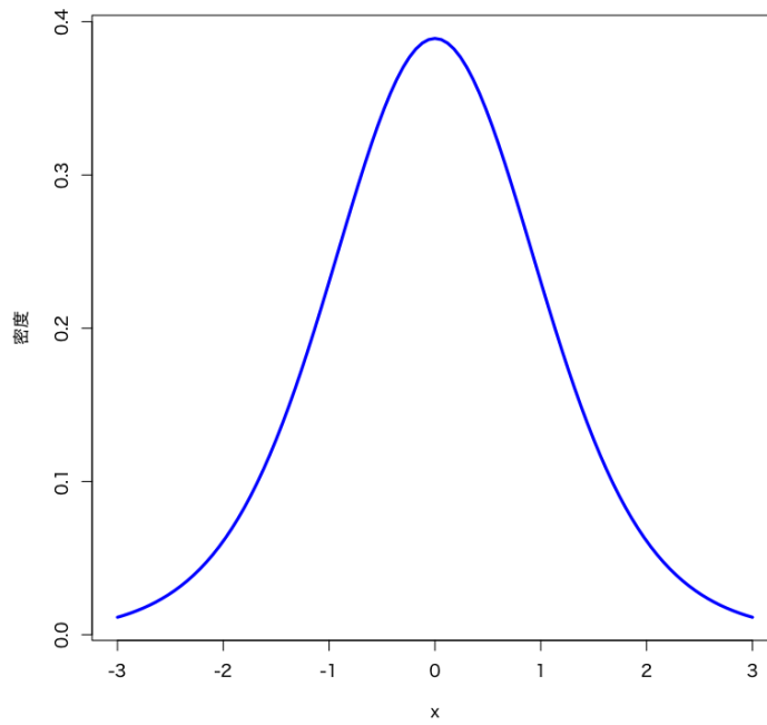
t-分布 (自由度 10; 歪度0, 超過尖度1)
