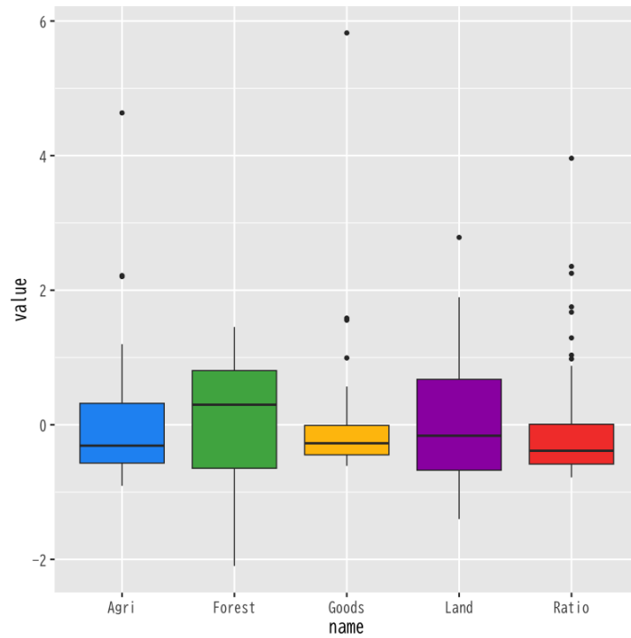
図 4: 箱ひげ図 (データを正規化)
