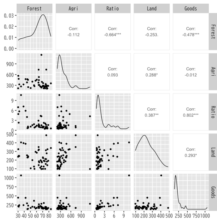
图 2: 散布图
