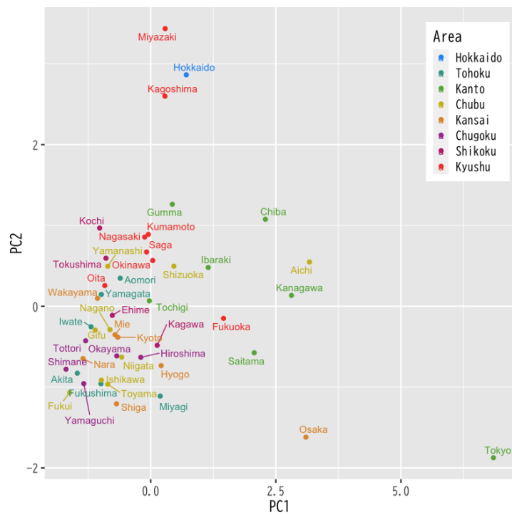
図 5: 主成分得点による散布図
