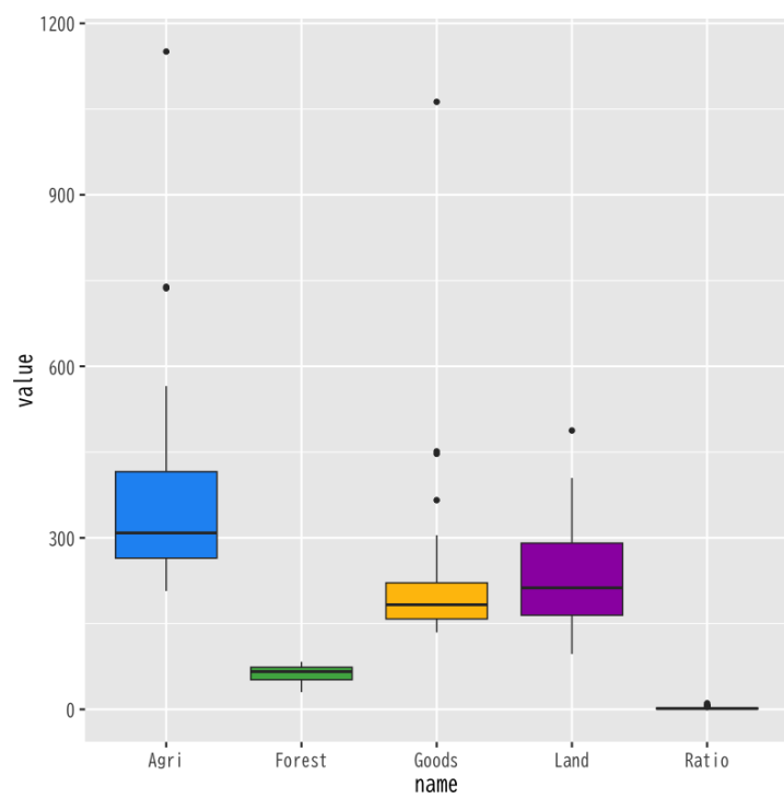
图 3: 箱ひげ图
